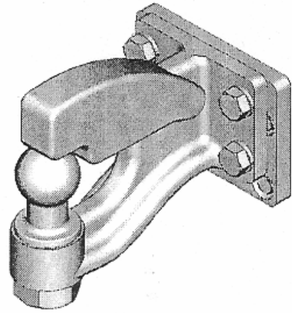
Pintle/2" Ball Hitch
